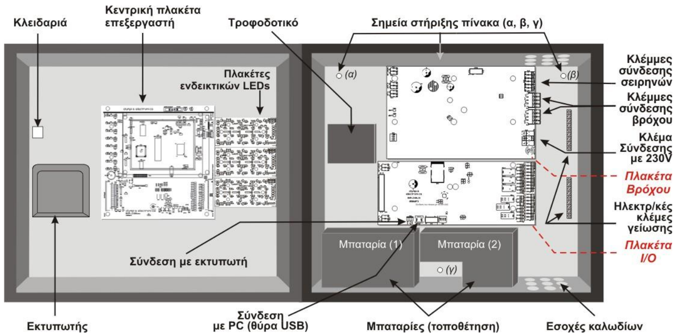
Σχήμα 3-1. Εσωτερικό πίνακα
