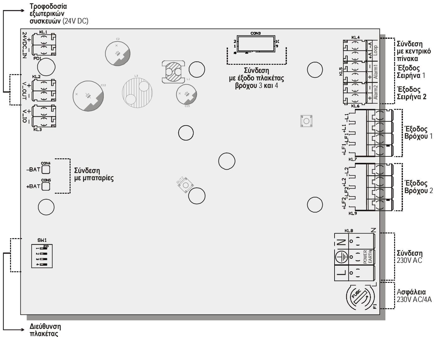
Σχήμα 3-2. Πλακέτα βρόχου
