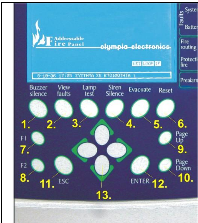
Σχήμα 1-2. Πληκτρολόγιο πίνακα
