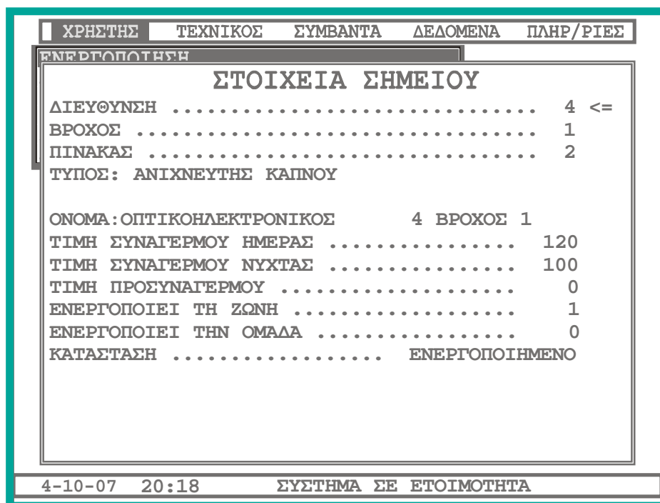
Σχήμα 4-8. Ιδιότητες σημείου
